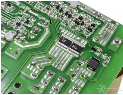
Particolare dei due Shunt utili per la rilevazione della corrente d'ingresso.
