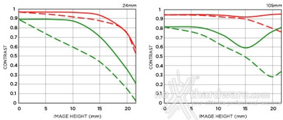
Sigma 24-105mm f/4 DG OS HSM , grafici MTF in posizione grandangolare e tele:
