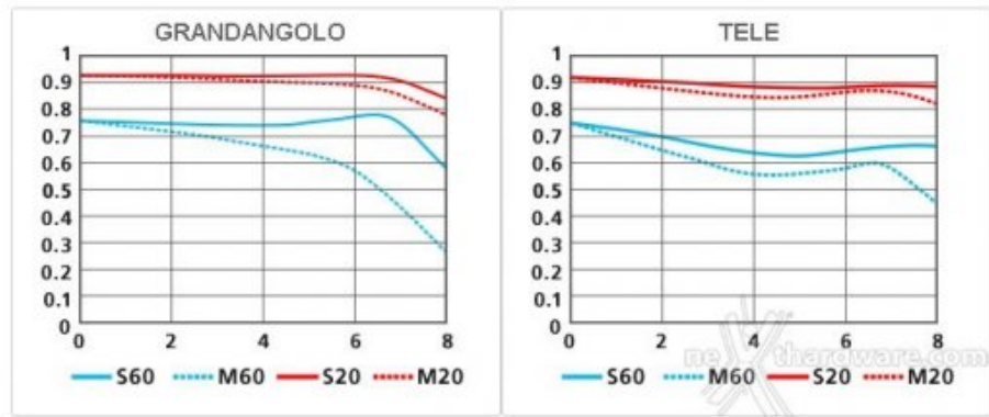
Obiettivo 1 Nikkor 11-27.5 F3.5-5.6, schema ottico e grafici MTF wide/tele
